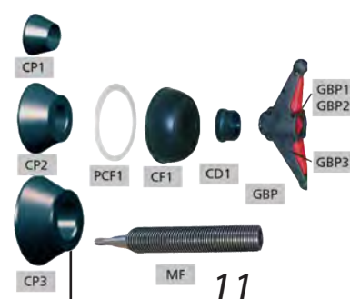
FBC EVO ZESTAW CENTRUJĄCO-MOCUJĄCY
